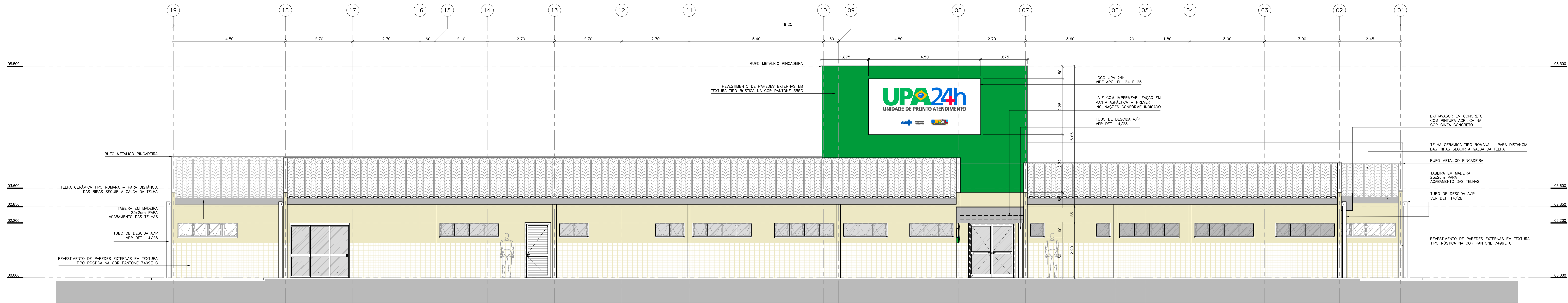
01 UNIDADE DE PRONTO ATENDIMENTO – PORTE 2 FACHADA 03 ESCALA: 1:50
